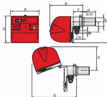
Rozměry hořáku
