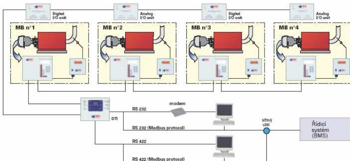
Příklad vysokoúrovňového zapojení I/O analogových modulů a kontrolního řídicího systému
