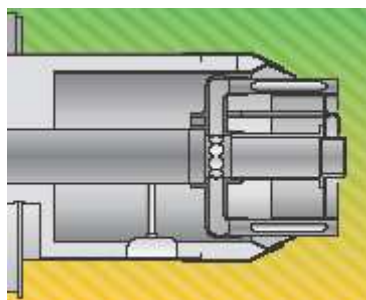
Příklad spalovací hlavy hořáků MODUBLOC MB LE
