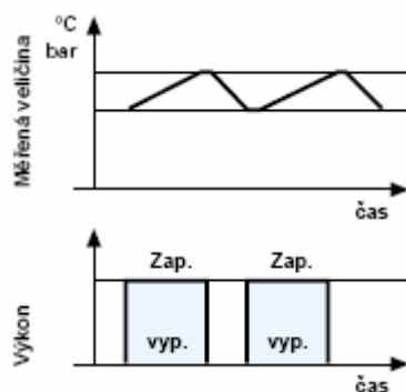
Jednostupňový provoz
