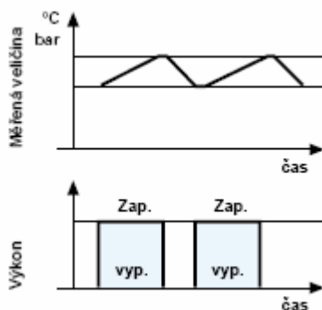
Jednostupňový provoz
