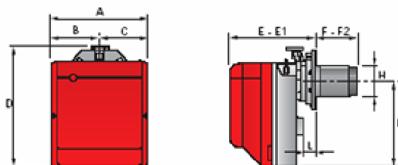
Rozměry hořáku
